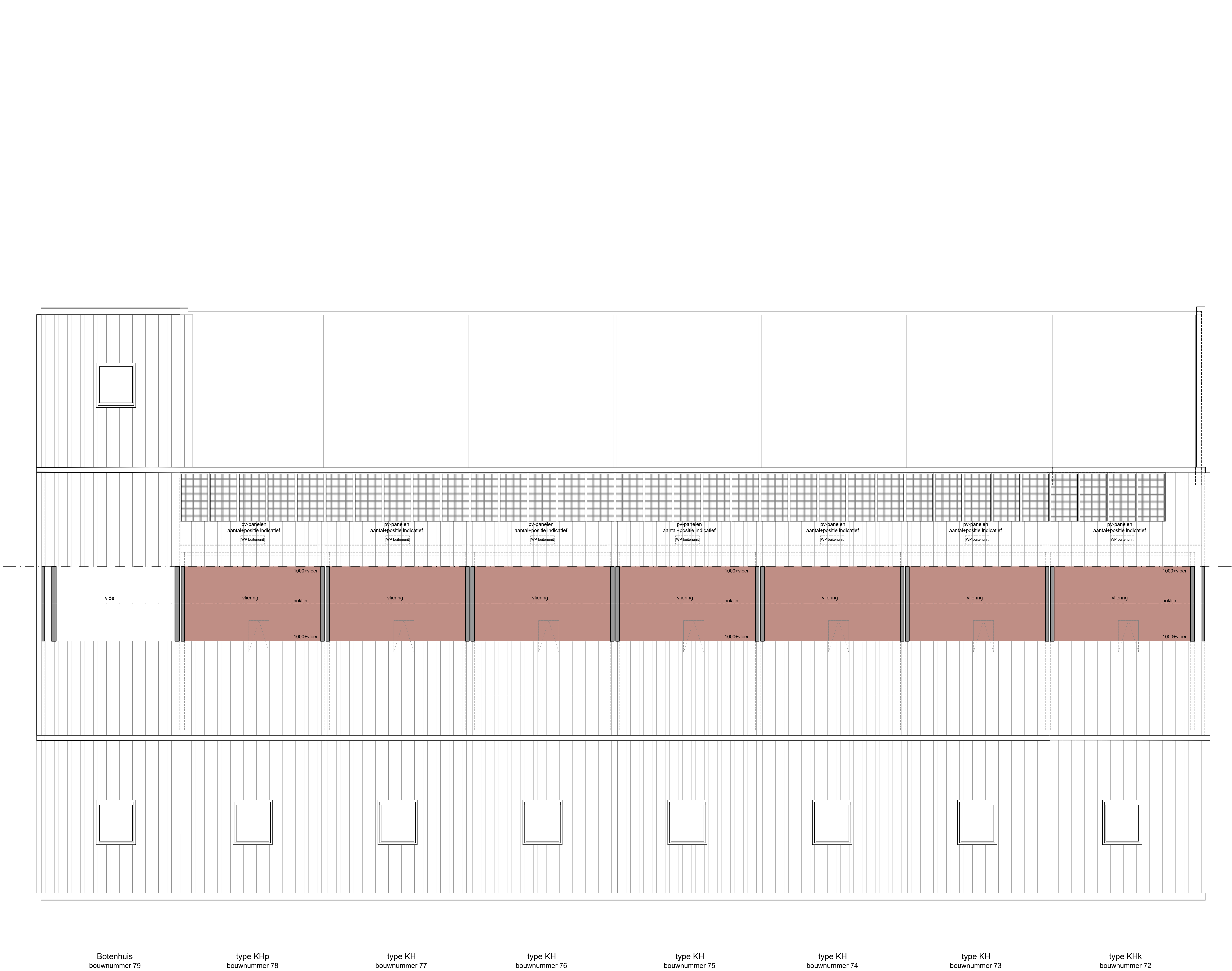
Vliering 1:50
