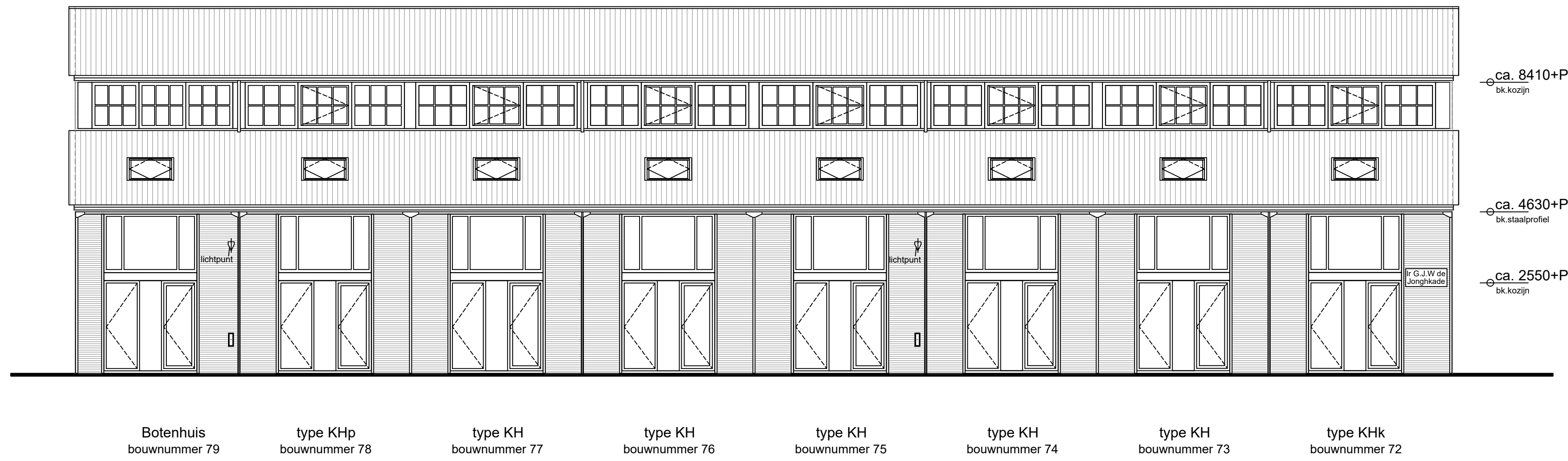
Voorgevel 1:100
