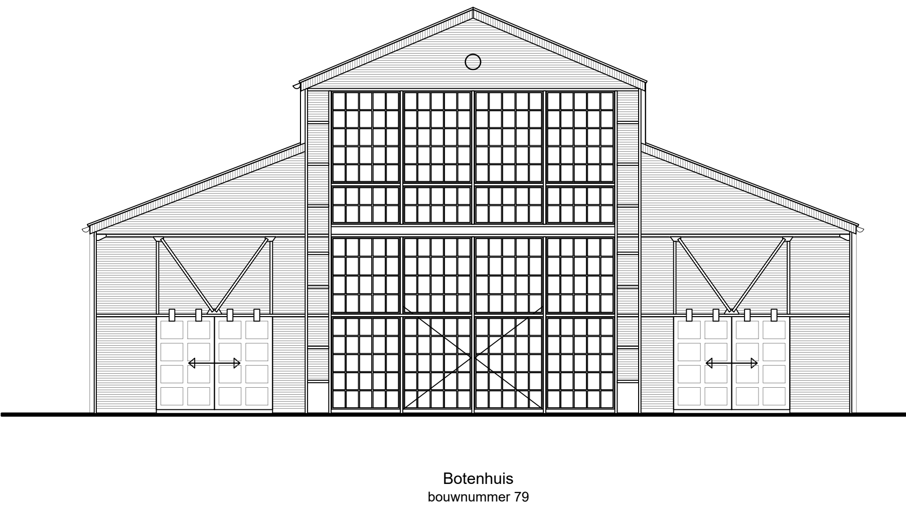
Kopgevel links 1:100
