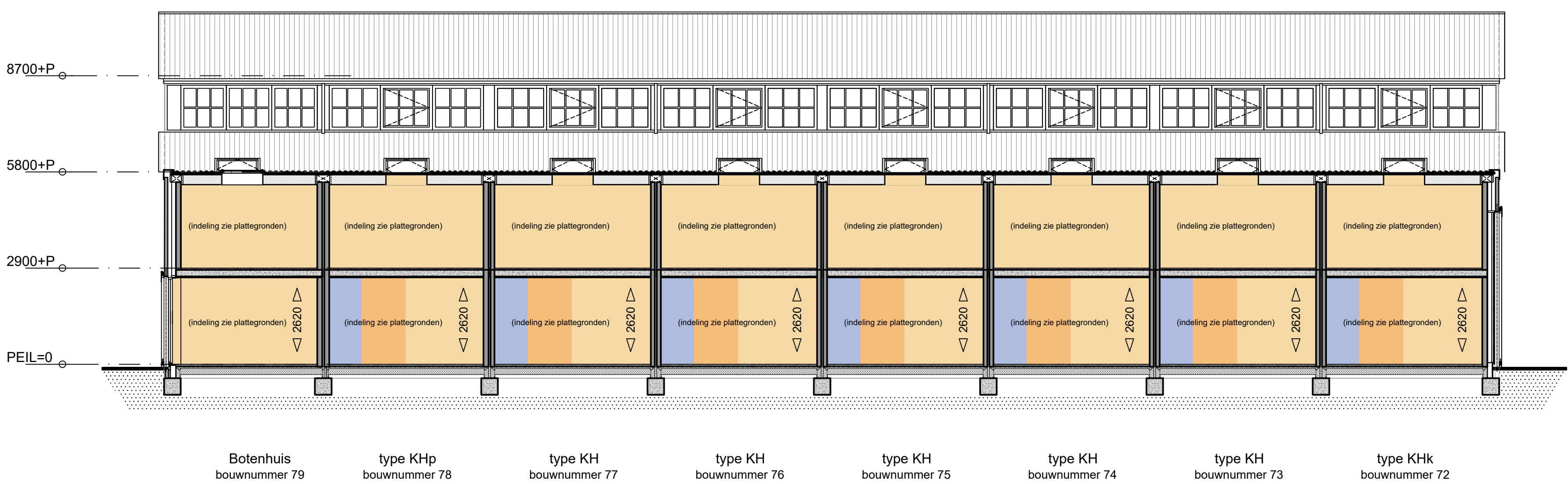
Langsdoorsnede 1:100
