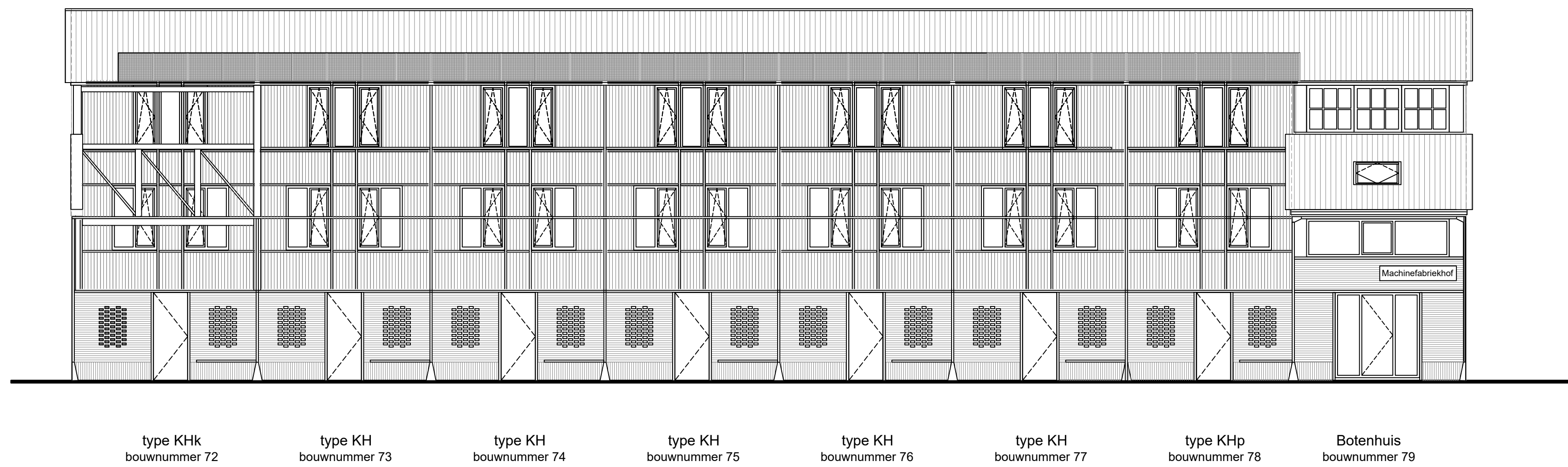
Achtergevel 1:100
