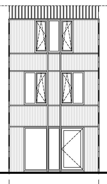
Fragment achtergevel 1:100
