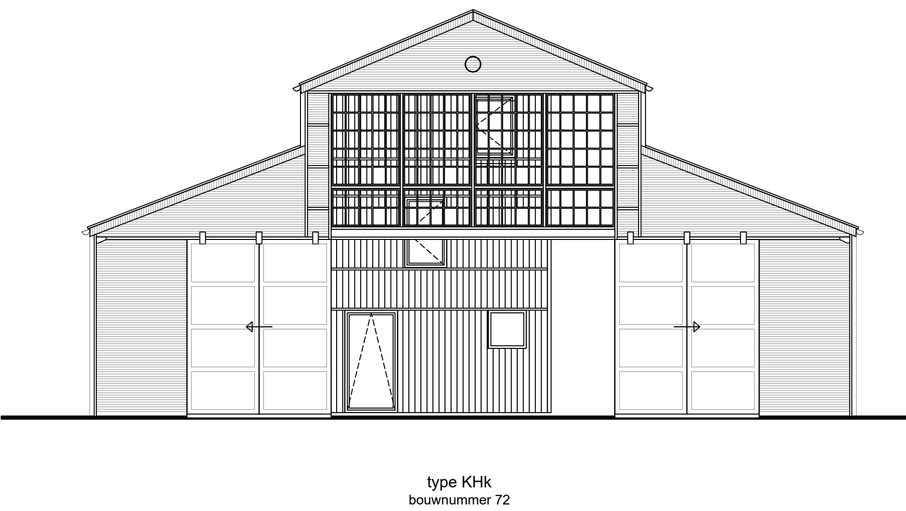
Kopgevel rechts 1:100
