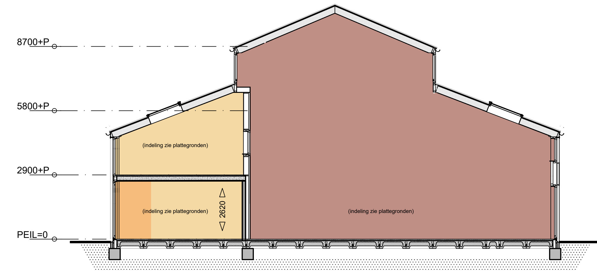
Dwarsdoorsnede 1:100
