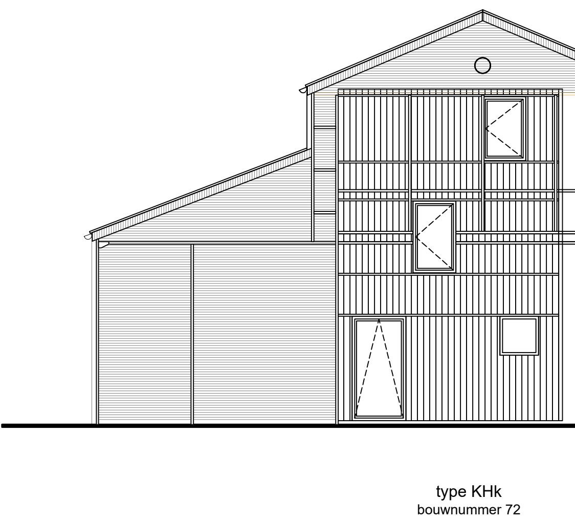
Fragment kopgevel rechts 1:100
