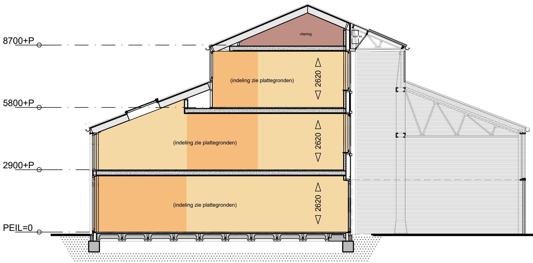
Dwarsdoorsnede 1:100
